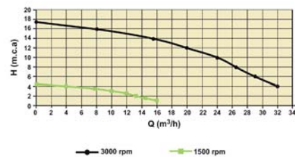
Curvas de rendimiento hidr ulico Hydraulic performance curves Courbes de performances hydrauliques Curve delle prestazioni idrauliche
