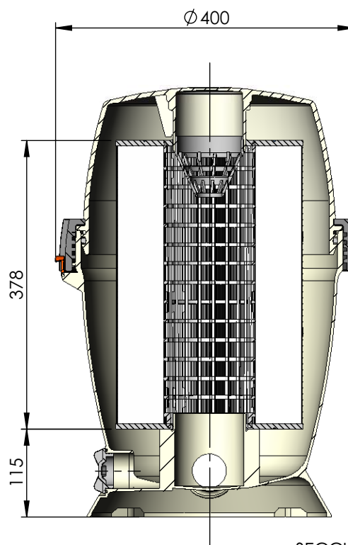
SECCIÓN D-D
