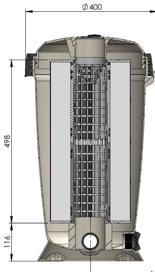
SECCIÓN D-D
