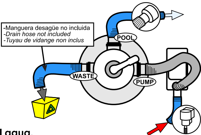
Circuito del agua. Circuit water. Circuit d'eau.
